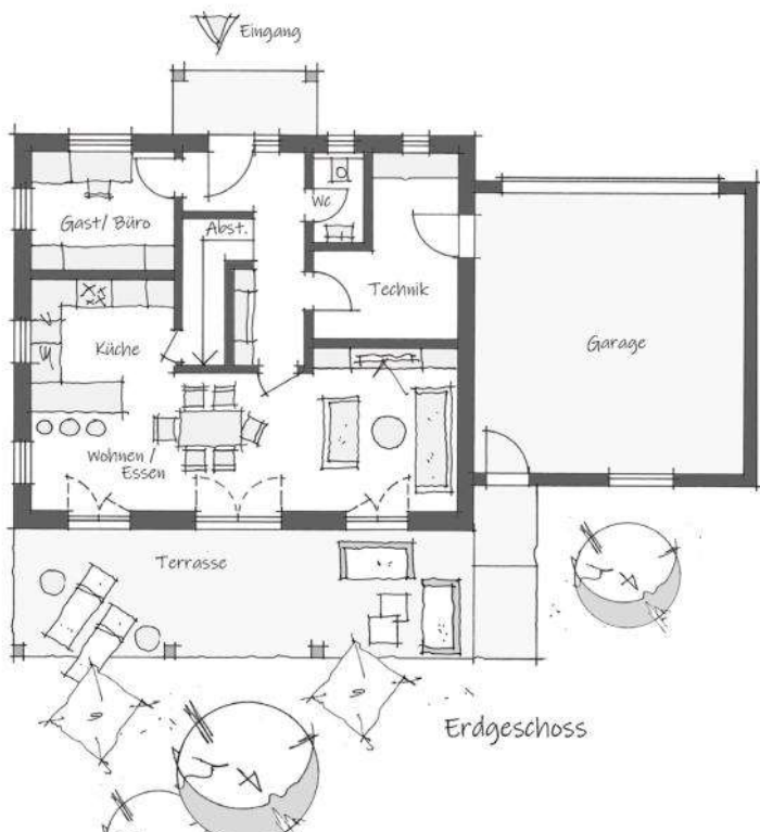
Grundrisse Kein Maßstab
